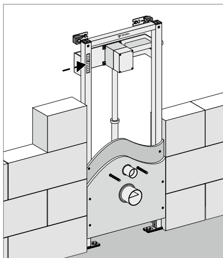
Montaggio davanti a una parete massiccia Costruzioni da murare
