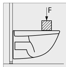
Prova a carico WC 400 kg Nel rispetto della norma DIN EN 997
