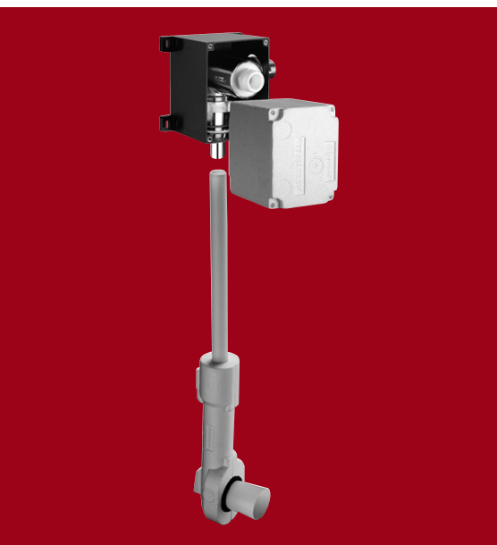
Sciacquone sottotraccia per WC COMPACT II
