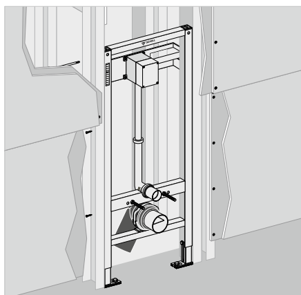
Montaggio su base a telaio Costruzioni a secco
